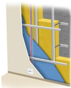
Ossature rapportée
